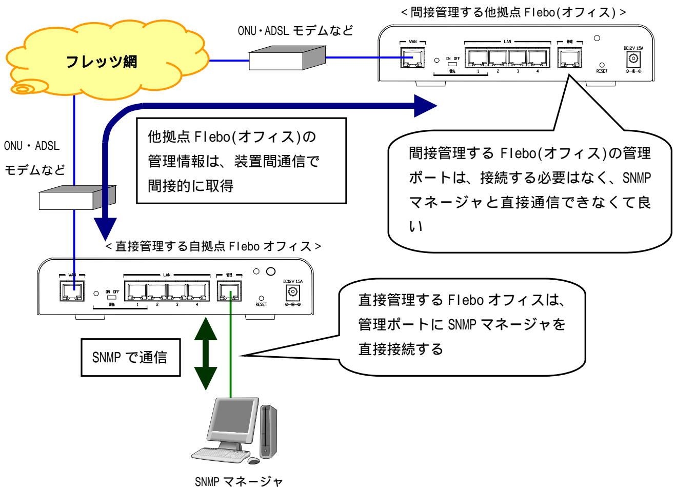
図 3.1.1 他拠点 Flebo(オフィス)を間接的に管理する場合
